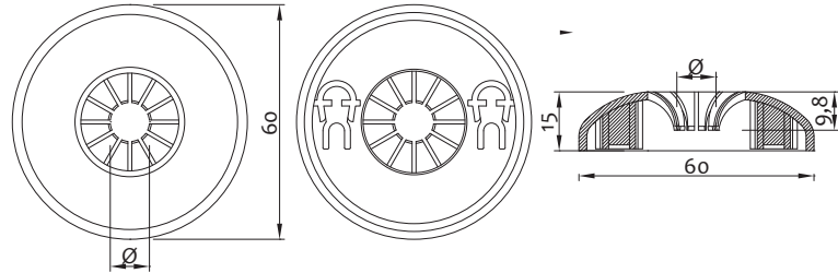
Rozetă universală cromată din ABS Chromed universal rosette
