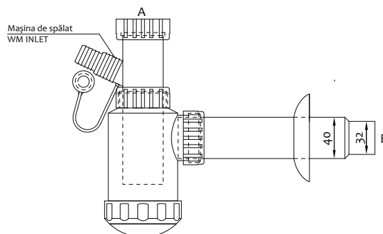
Sifon chiuvetă cu scurgere pentru mașina de spălat Bottle trap for single sink
