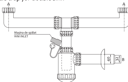
Sifon chiuvetă dublă cu scurgere pentru mașina de spălat Bottle trap for double sink
